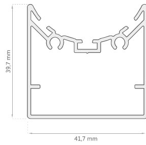
Marco Fijo D-2013
