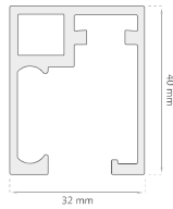
Expansor D-2085
