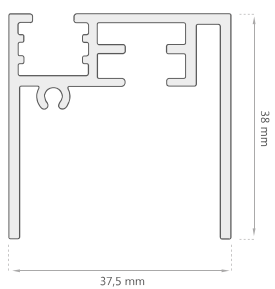
Esquinero F.L. D-2102
