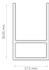
Marco Fijo F.L. Corto K-0304/8
