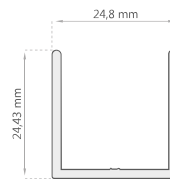
Marco Fijo Corto K-0304
