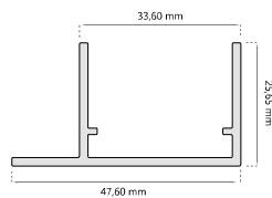
Expansor D-2112
