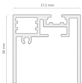
Marco F.L. D-2099
