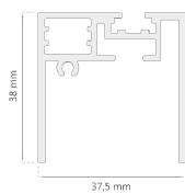
Marco Fijo D-2107
