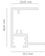
Marco D-2072
