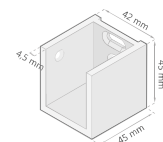
SOPORTE GUÍA DERECHO
