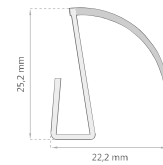
PGE-1100
