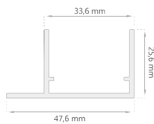
Expansor D-2112
