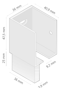
Soporte Guía Pared Izquierdo
