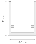
Marco Fijo D-2107
