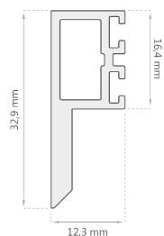
Expansor Marco Fijo Corto J-1110
