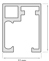
Guía Superior D-2075
