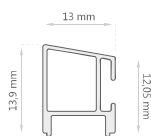
Perfil Base D-2091
