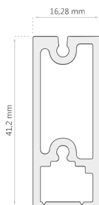
Guía D-2106
