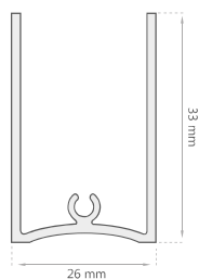
Marco D-2072
