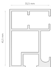
Marco Fijo D-2080
