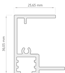
Esquinero F.L. D-2102
