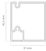
Marco esquinero D-2108
