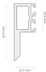
Tapa Marco D-2077
