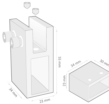
Conjunto Soporte Vidrio Techo
