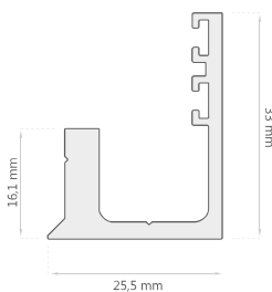
Perfil Base D-2091
