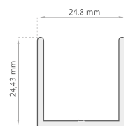
Marco Fijo Cierre Corto K-0304/6
