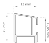
Perfil Base D-2091
