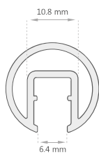
Expansor Marco Fijo Corto J-1110
