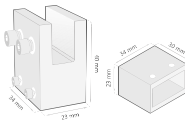
Ángulo Cogida Pared
