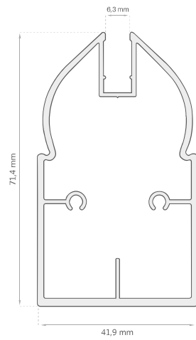
Marco Fijo D-2013
