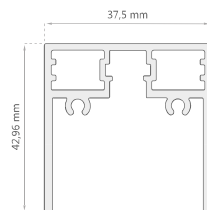
Marco Lateral 2 Hojas Correderas D-2117
