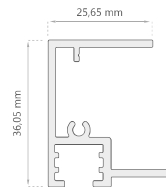
Esquinero F.L. D-2102
