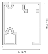
Guía Superior Cerrada D-2096
