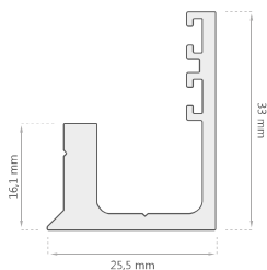
Tapa Marco D-2077
