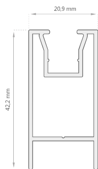
Marco Fijo D-2029
