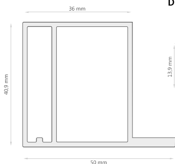
Marco Cierre D-2081
