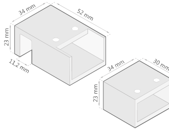
Conjunto Soporte Vidrio Tubo
