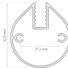
Tubo Autorretornable D-2034
