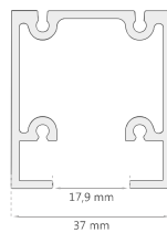
Guía Superior 2 Hojas Correderas D-2116
