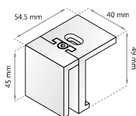
Ángulo Central Regulable
