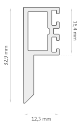
Marco Cierre D-2081
