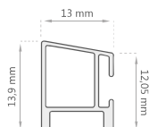
Marco D-2072
