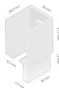
Tapa Marco D-2077
