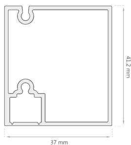
Guía D-2106
