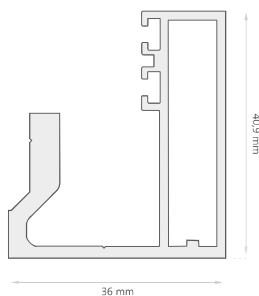
Marco Fijo D-2076
