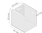
SOPORTE GUÍA IZQUIERDO
