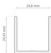
Expansor Marco Fijo Corto J-1110
