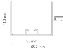
Guía Superior D-2065
