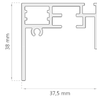
Marco Imán D-2100
