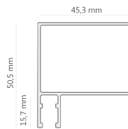
Esquinero F.L. D-2054
