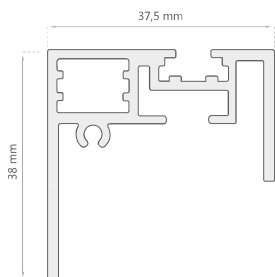
Marco Fijo D-2107
